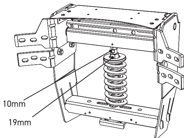
ALTERNATIEF SCHARNIER
