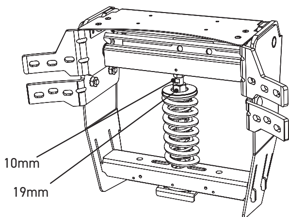
ALTERNATIV HINGE
